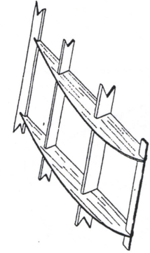
starba křídla
